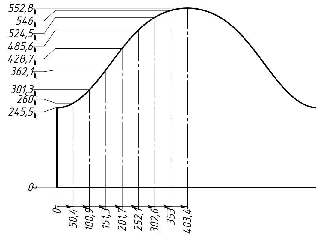
Поз.2 (Патрудок) развертка
